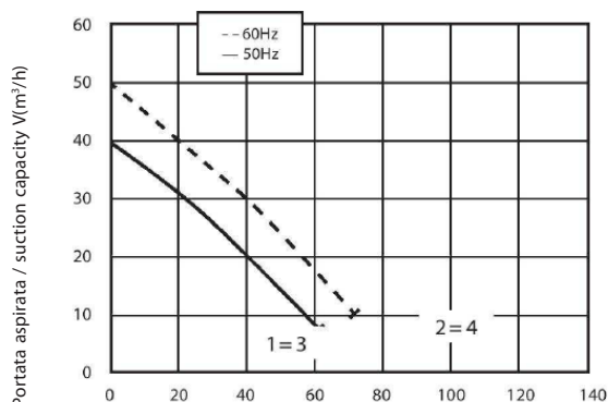
ASPIRAZIONE / EXHAUST
