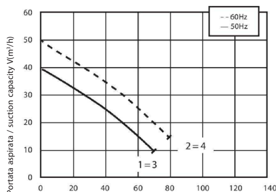
COMPRESSIONE / COMPRESSION
