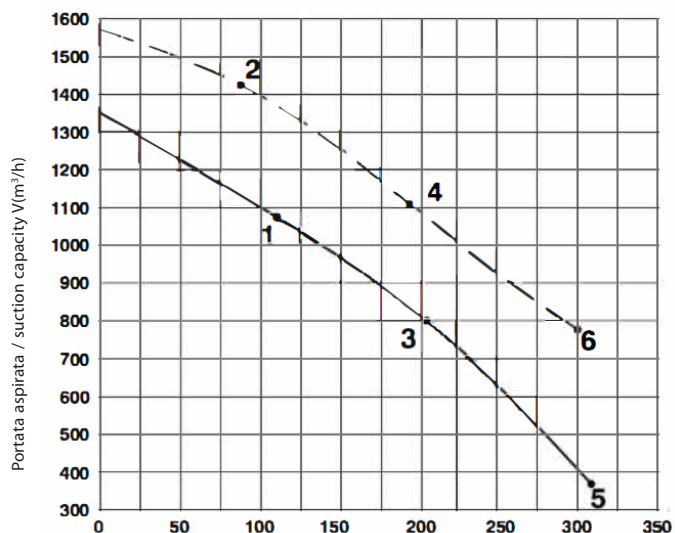
ASPIRAZIONE / EXHAUST
